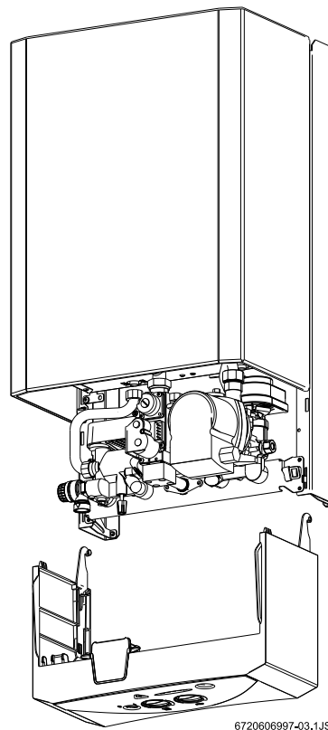
Fig. 9 Smontaggio del quadro comandi.
