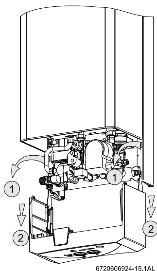
Fig. 23 Posizione di manutenzione per l'accesso ai componenti
