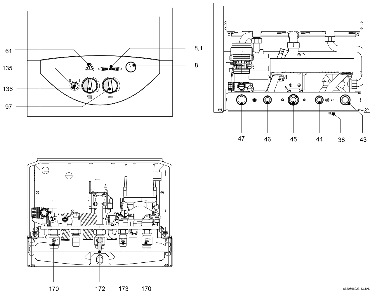
Fig. 15 Vista frontale, posteriore ed inferiore
