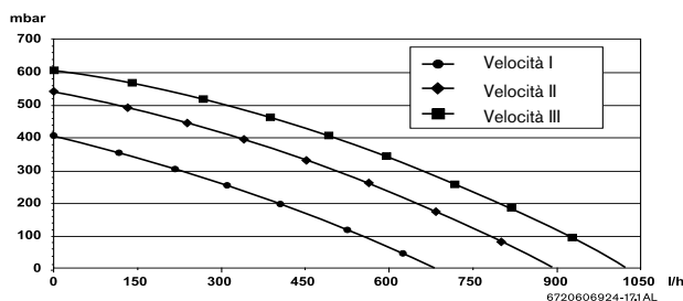
Fig. 5 Curva caratteristica del circolatore
