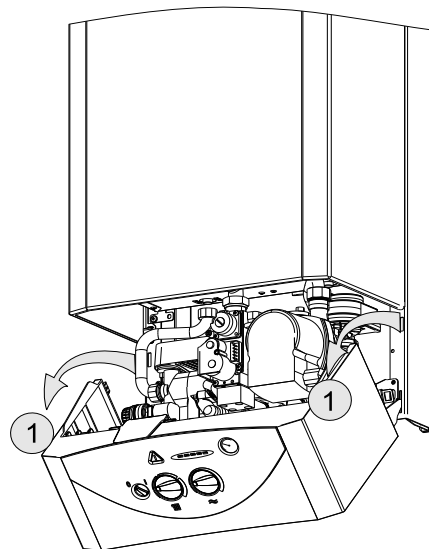
Fig. 20 Posizione di manutenzione
