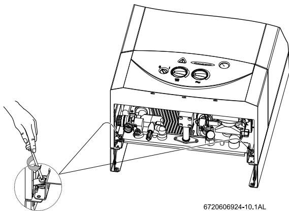
Fig. 7 Viti di fissaggio quadro comandi
