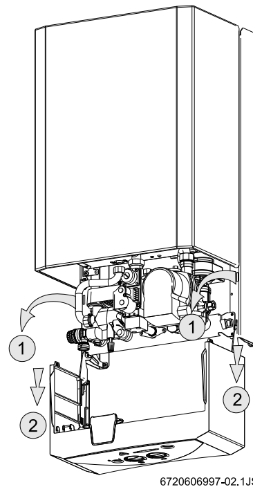
Fig. 8 Quadro comandi nella posizione di manutenzione.
